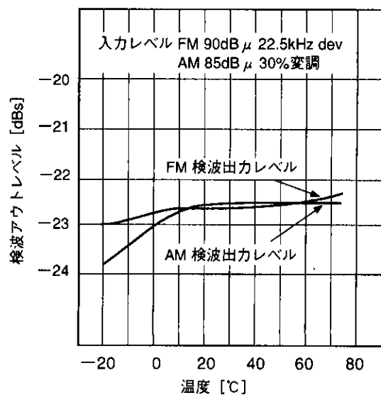
検波出力レベル温度特性
