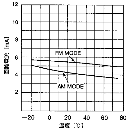
回路電流温度特性
